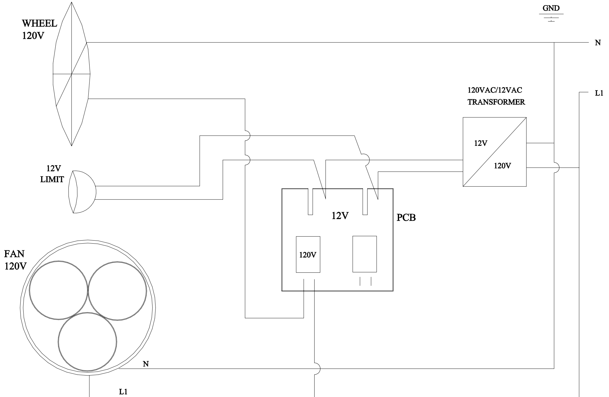
SMART SWITCH 120V FAN & WHEEL ; 12V LIGHT
