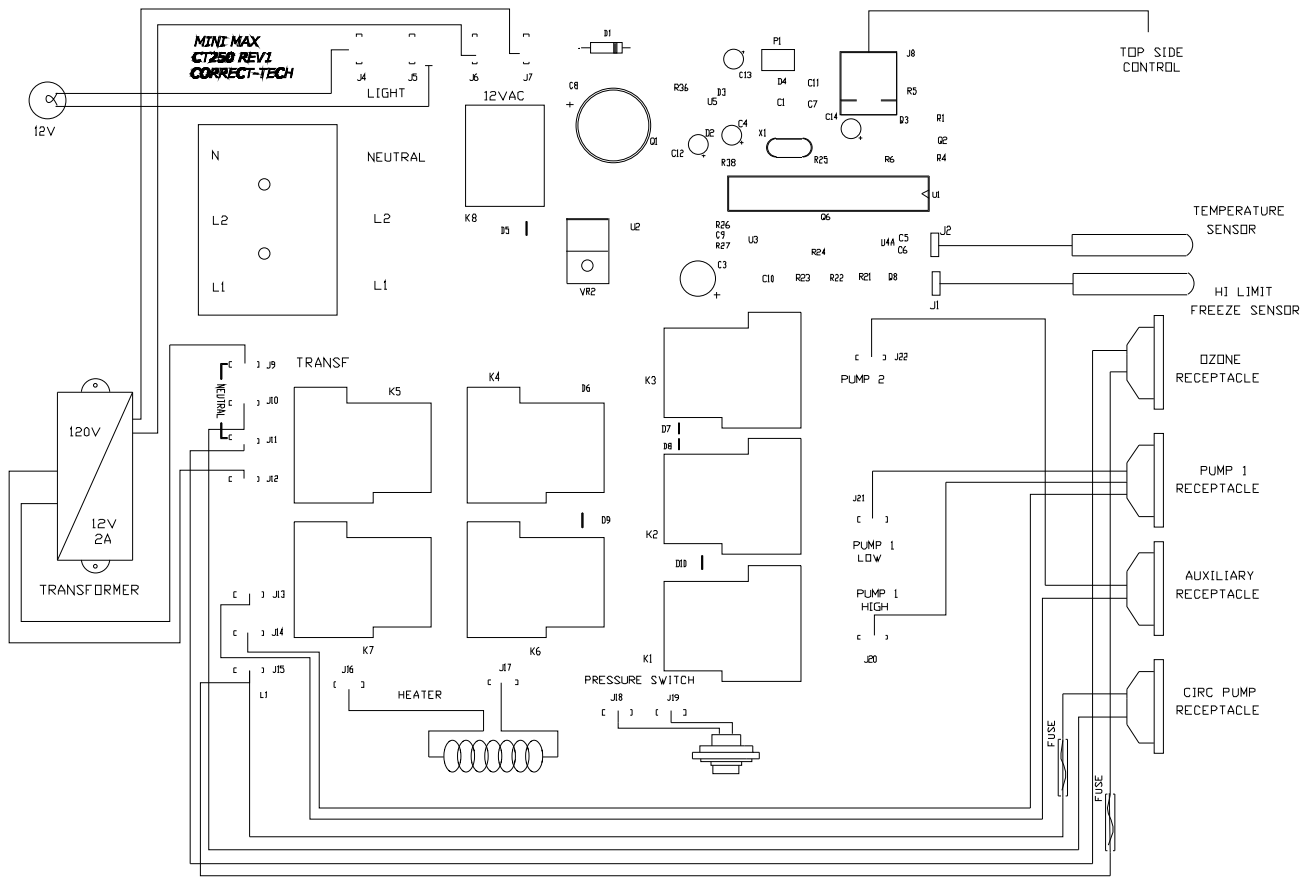
4-30-1806C - Mini Max Digital schematic
